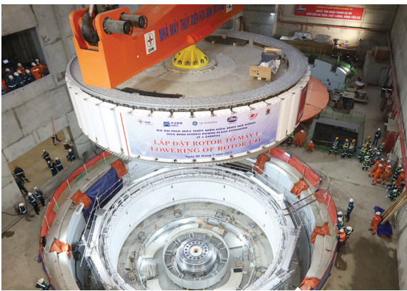
● Lắp đặt rotor tổ máy số 1. (Ảnh: Hà Trung)
